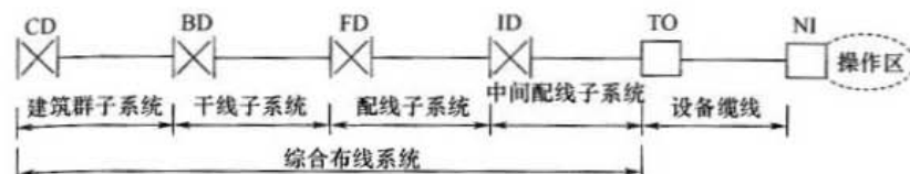
图 3.7.3 工业环境布线系统架构
