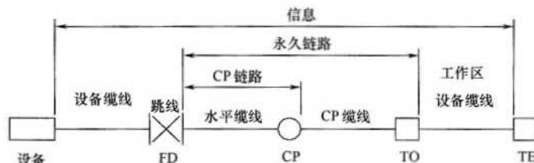
图 3.2.2 布线系统信道、永久链路、CP 链路构成
