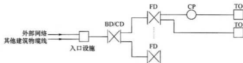
图 3.1.2-3 综合布线系统引入部分构成
