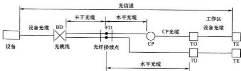
图 3.2.4-2 光纤信道构成 2
